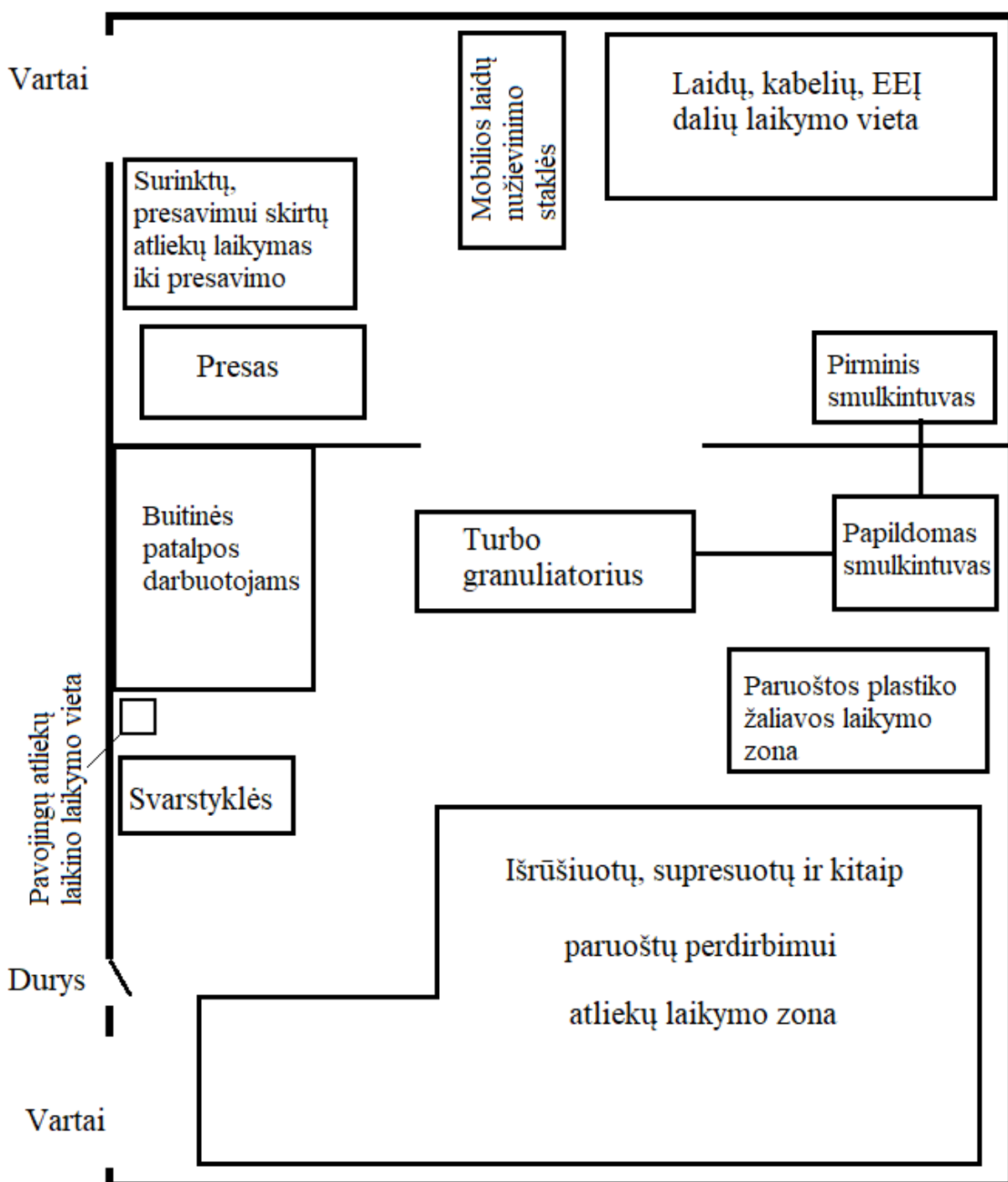
3 schema. Patalpų naudojimo, atliekų laikymo zonų schema.
