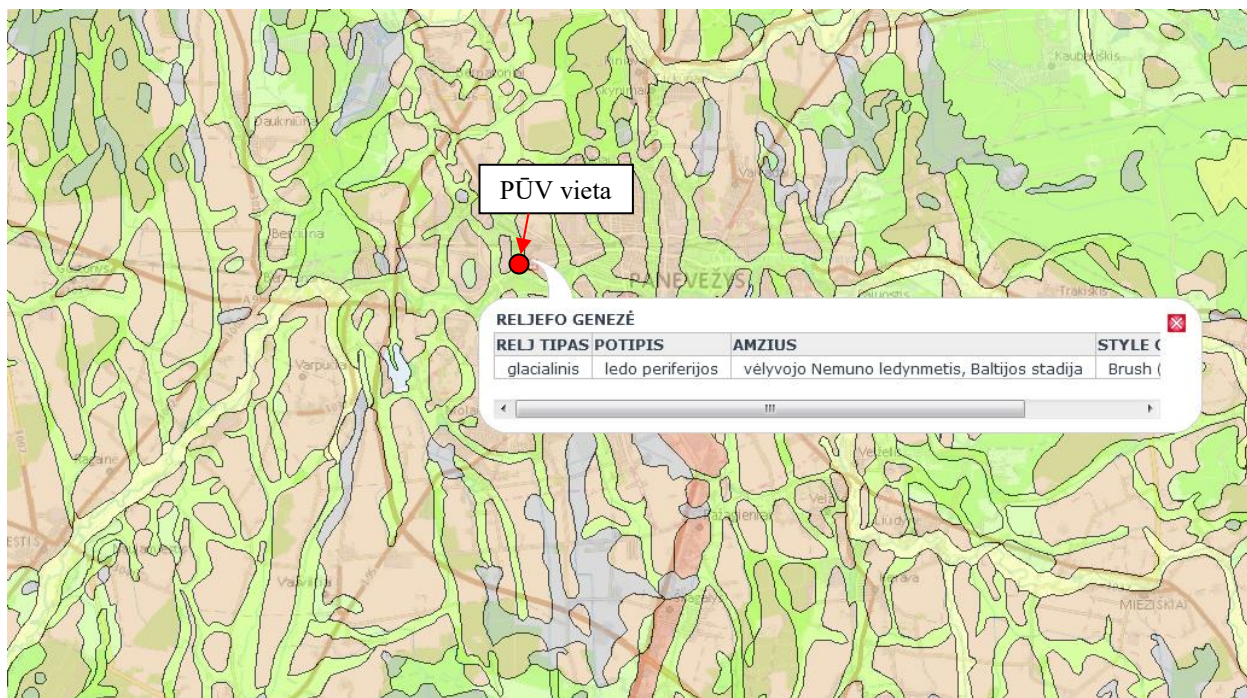
7 pav. Ištrauka iš Lietuvos geomorfologinio žemėlapiu (inf.šaltinis – www.lgt.lt/epaslaugos/ )
